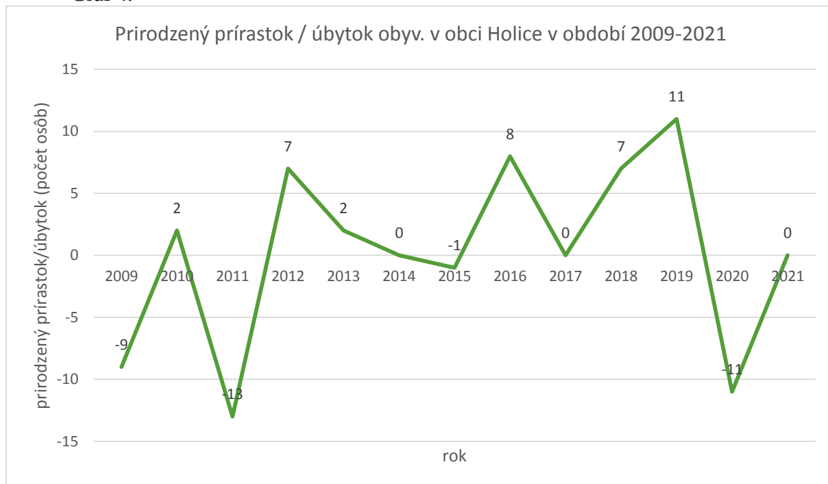
Graf 4:
